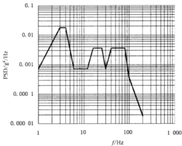
图 8 钢板弹簧卡车的随机振动功率谱曲线
