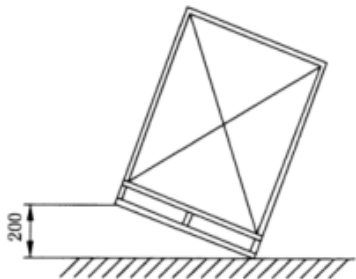
图 4 旋转面跌落试验
