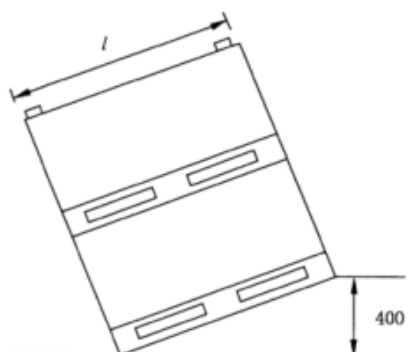
图7 堆码稳定性试验示意图
