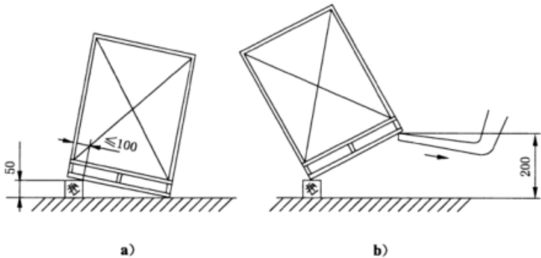
图 5 旋转跌落棱或角冲击试验
